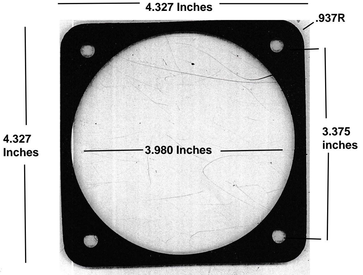
007 PANEL GASKET (3.2238.01)
