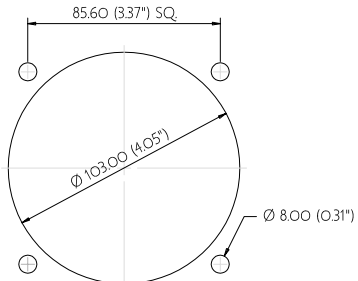
ANSI CUTOUT
