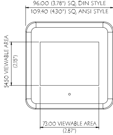
DIN CUTOUT
